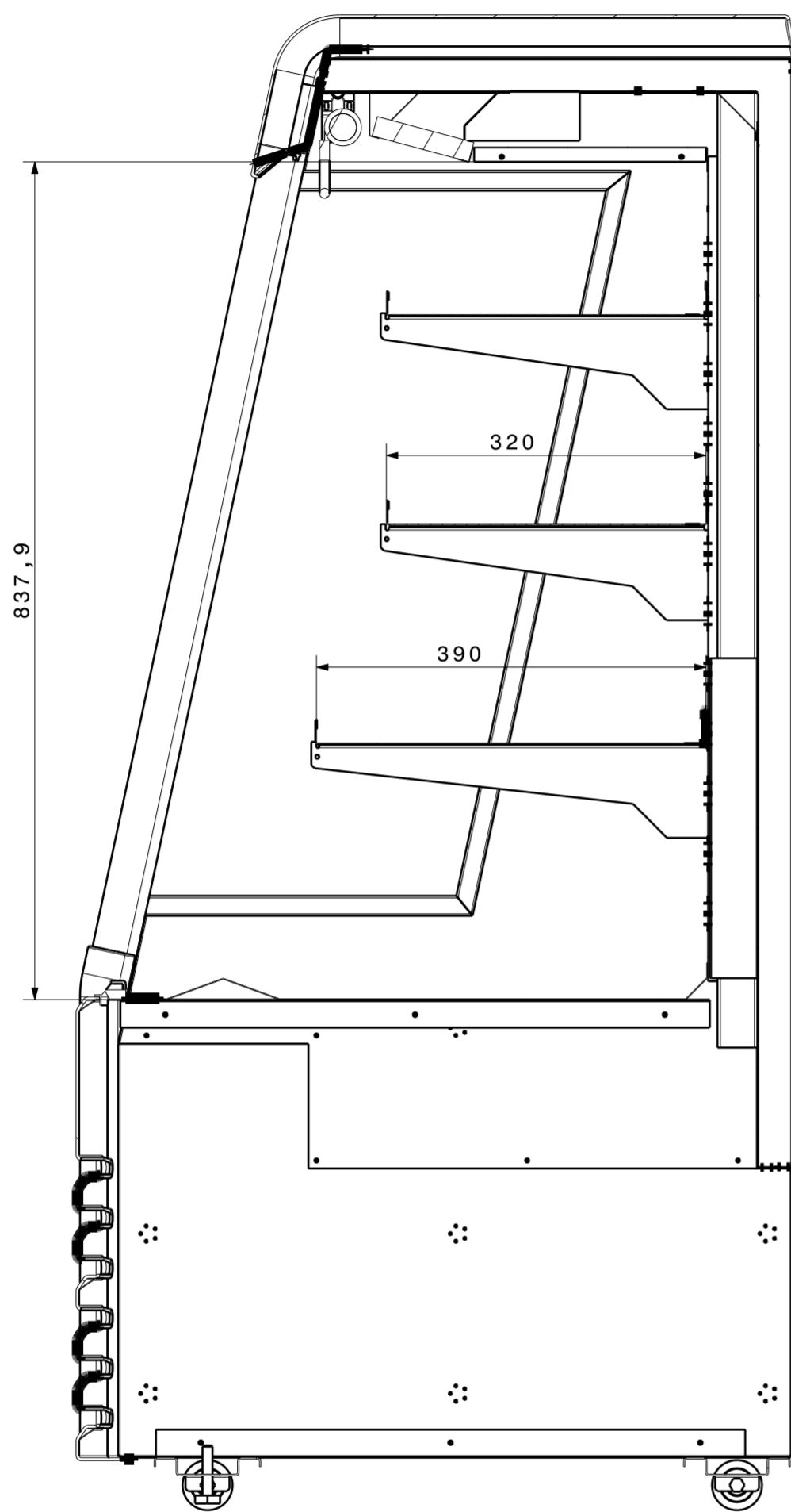
Schnitt A-A Maßstab: 1:6
